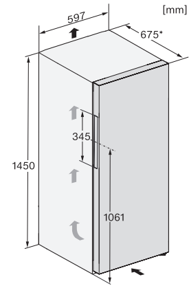
K4323FD, FN4322E, Aufstellskizze (*Fußnote) (Skizze)
